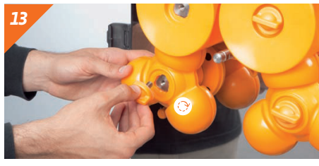
Schrauben Sie die Sicherheitsschrauben fest auf. Fehlende Schrauben müssen unbedingt ersetzt werden. Die Maschine niemals ohne alle Schrauben benutzen.
